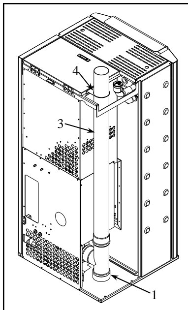
Uscita fumi sul lato superiore
