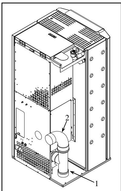
Uscita fumi sul lato posteriore
